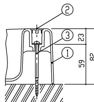
固定部詳細<1/3>
