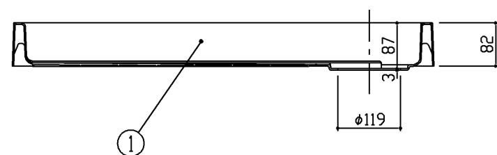
断面A-A
